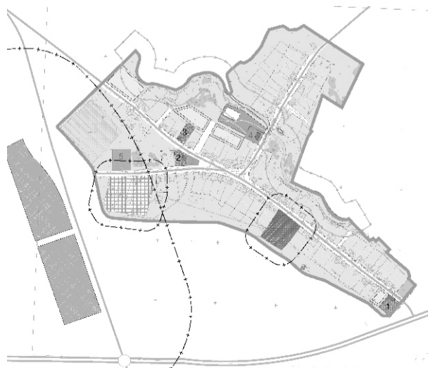
Схема генерального плана д. Маркова
