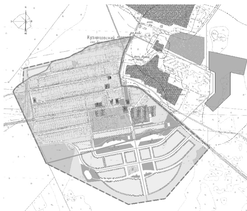
Схема генерального плана пос. Кузнецовский
